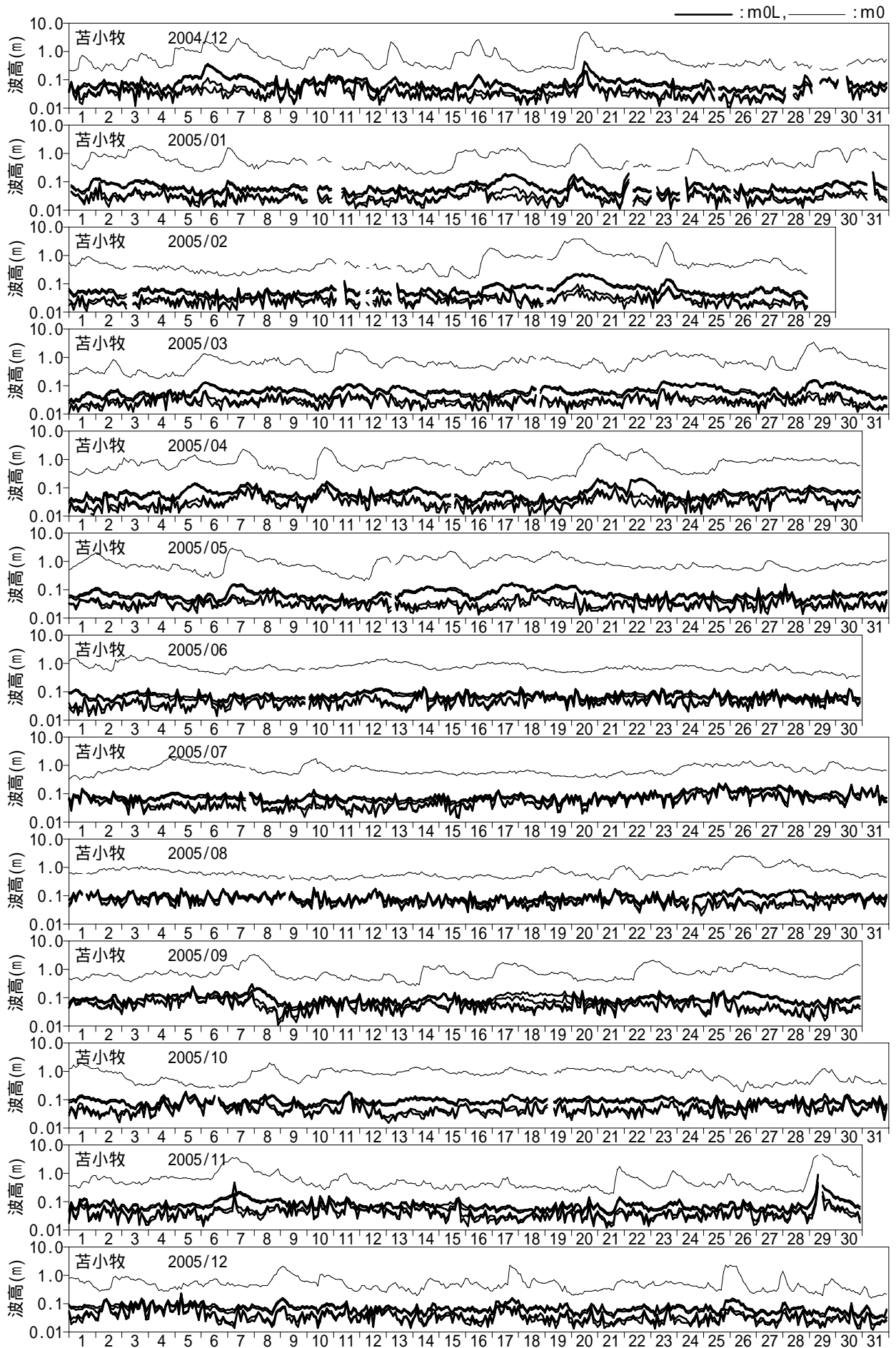
付図 - C.1.28 長周期波高の経時変化図 (苦小牧)
