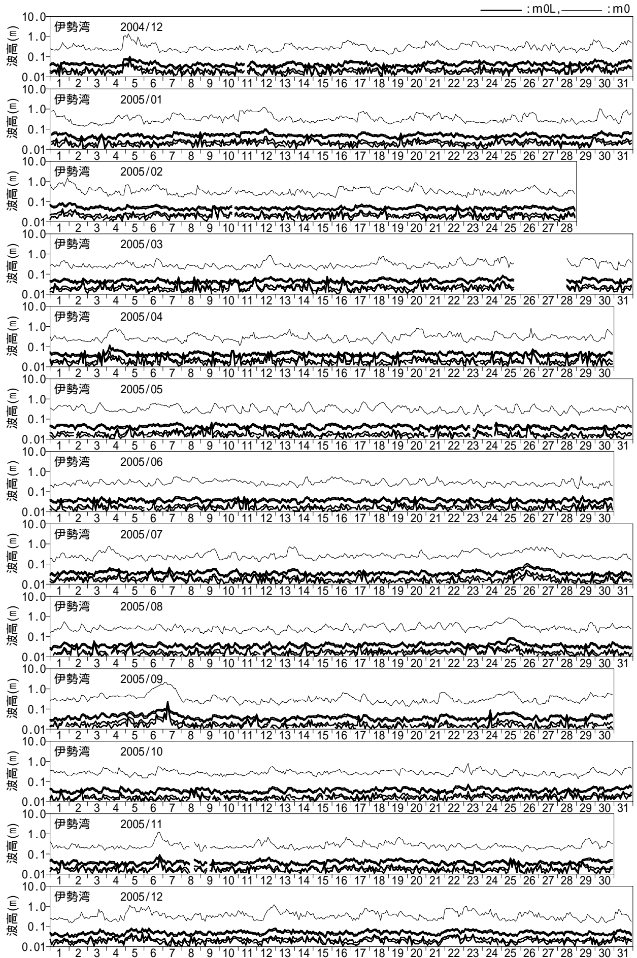
付図 - C.1.45 長周期波高の経時変化図 (伊勢湾)
