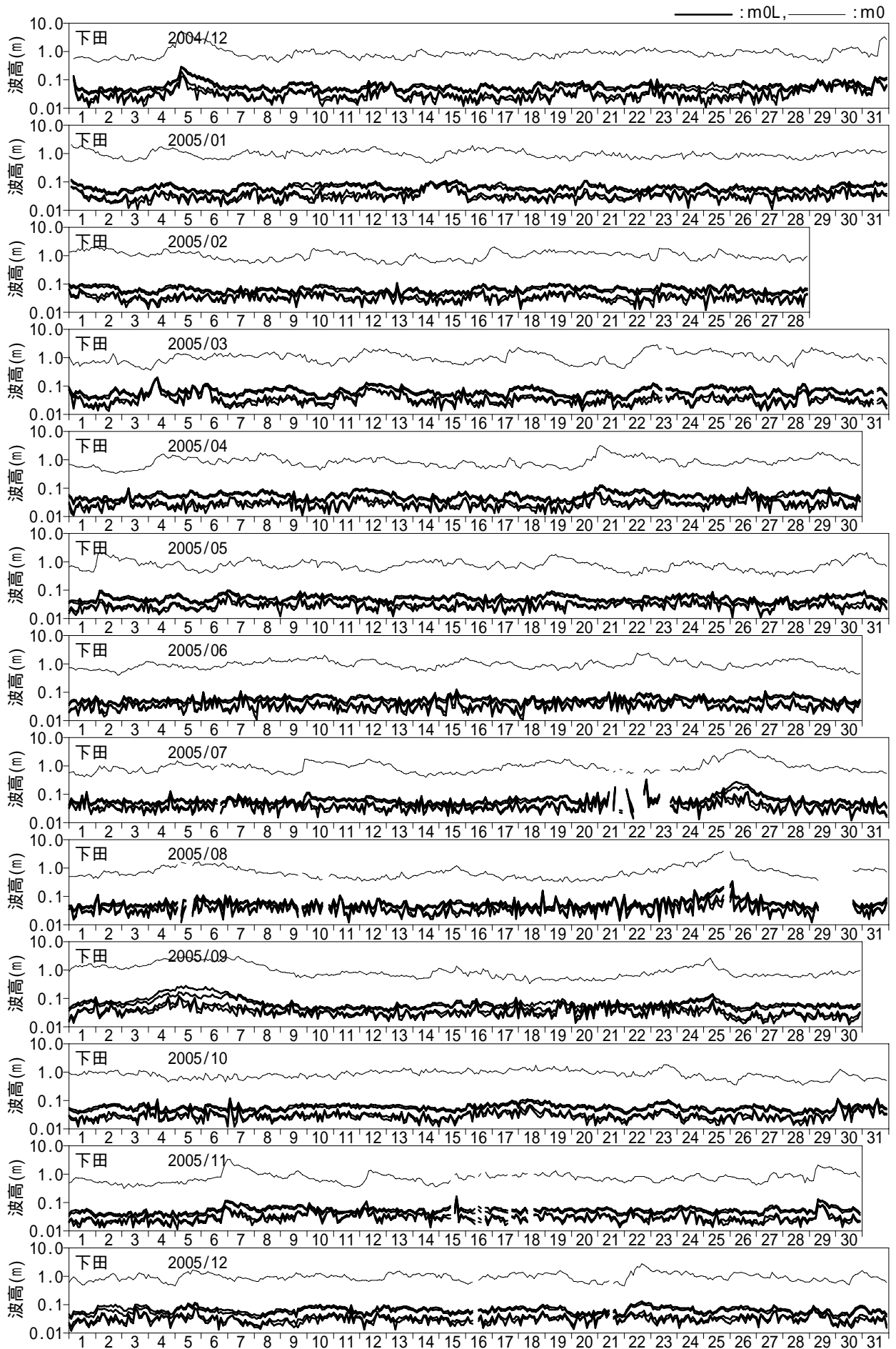
付図 - C.1.42 長周期波高の経時変化図 (下田)
