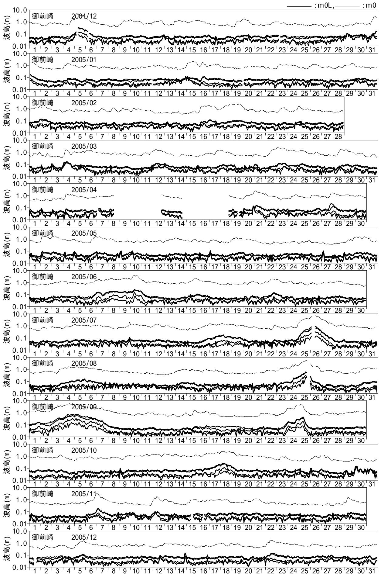
付図 - C.1.44 長周期波高の経時変化図 (御前崎)
