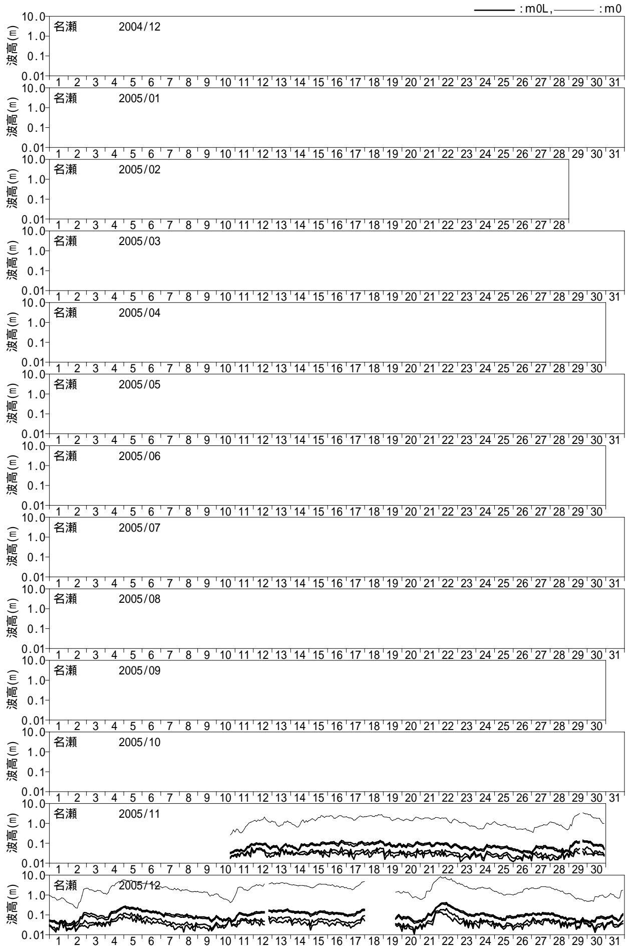
付図 - C.1.23 長周期波高の経時変化図 (名瀬)
