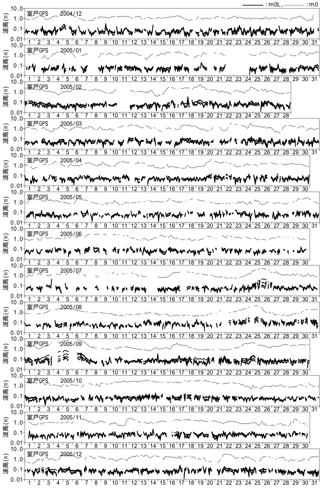
付図 - C.1.49 長周期波高の経時変化図 (室戸GPS)
