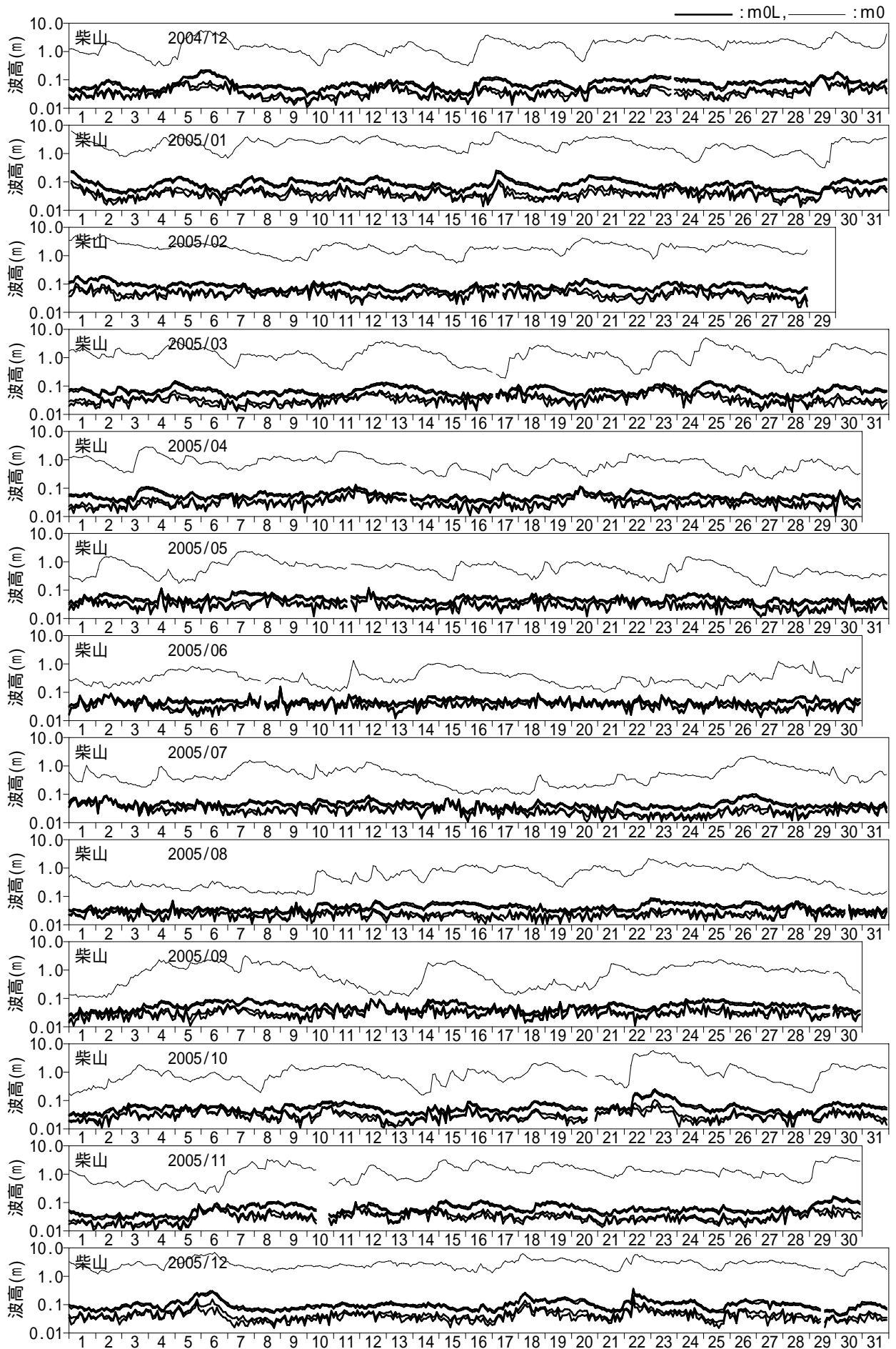
付図 - C.1.15 長周期波高の経時変化図 (柴山)
