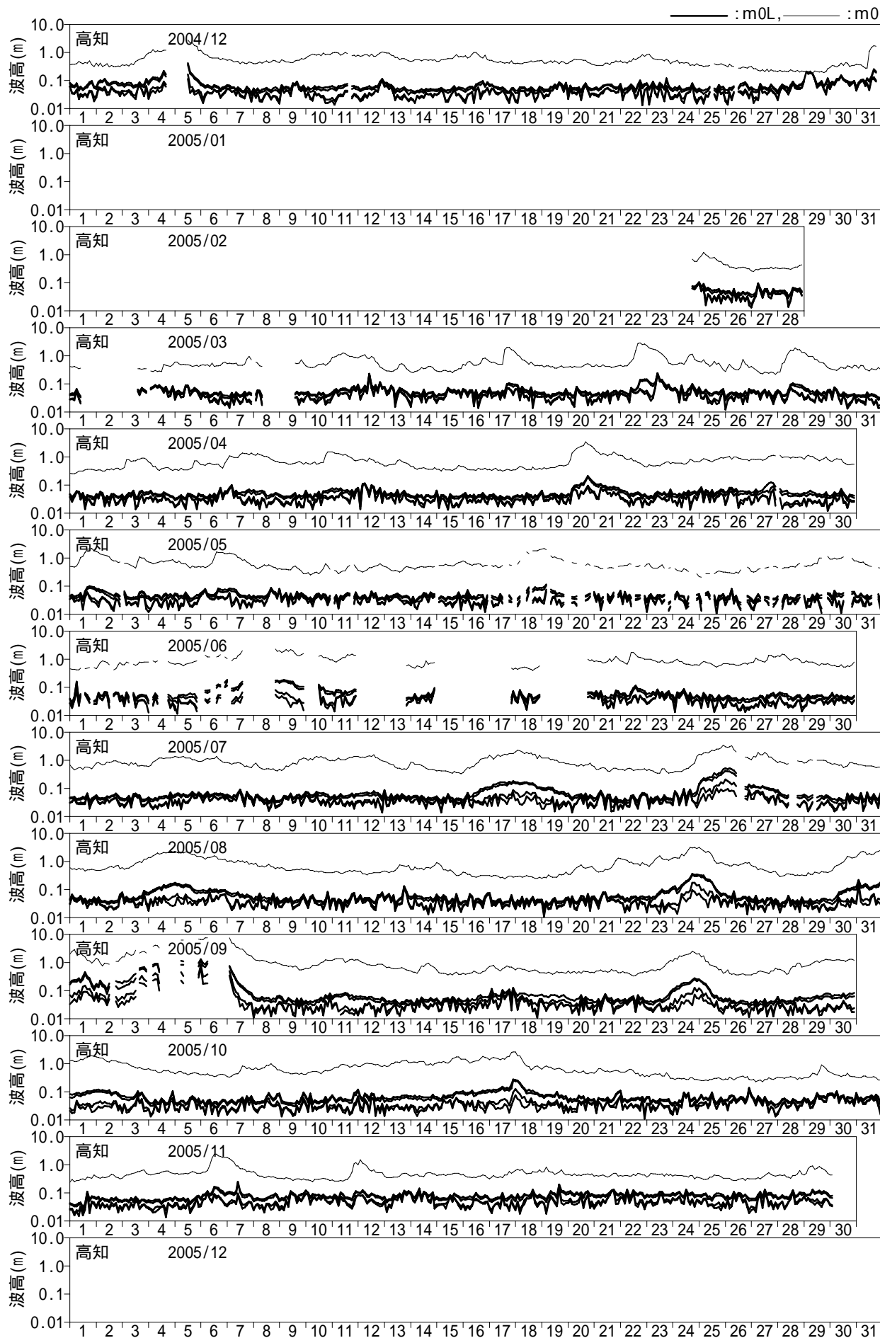
付図 - C.1.51 長周期波高の経時変化図 (高知)
