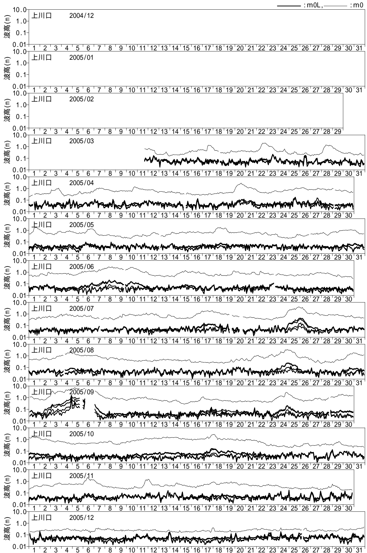
付図 - C.1.52 長周期波高の経時変化図 (上川口)
