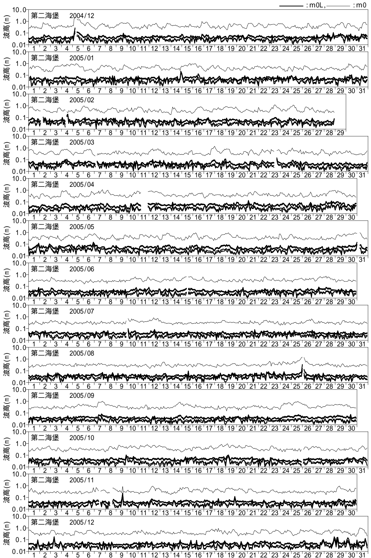
付図 - C.1.39 長周期波高の経時変化図 (第二海堡)
