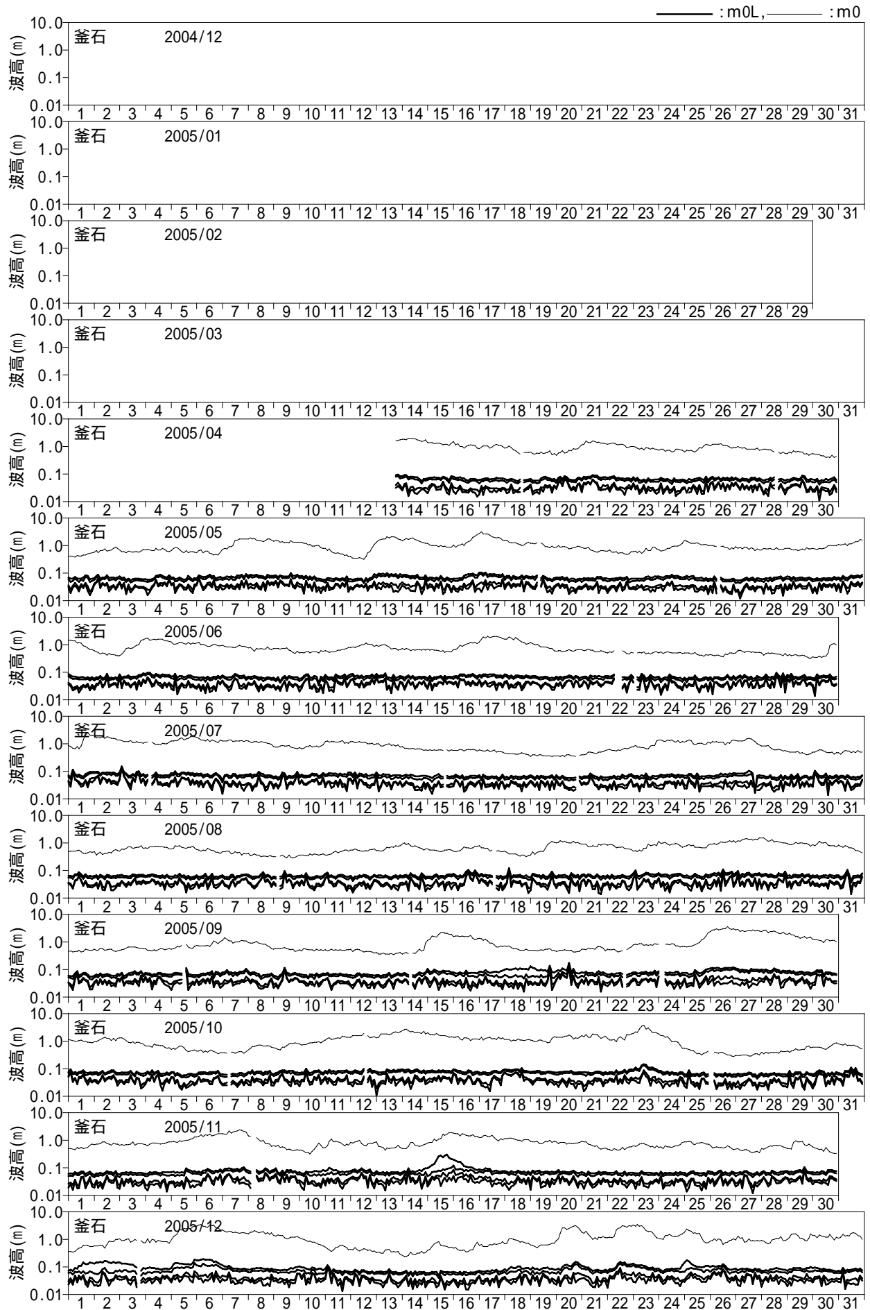
付図 - C.1.32 長周期波高の経時変化図 (釜石)
