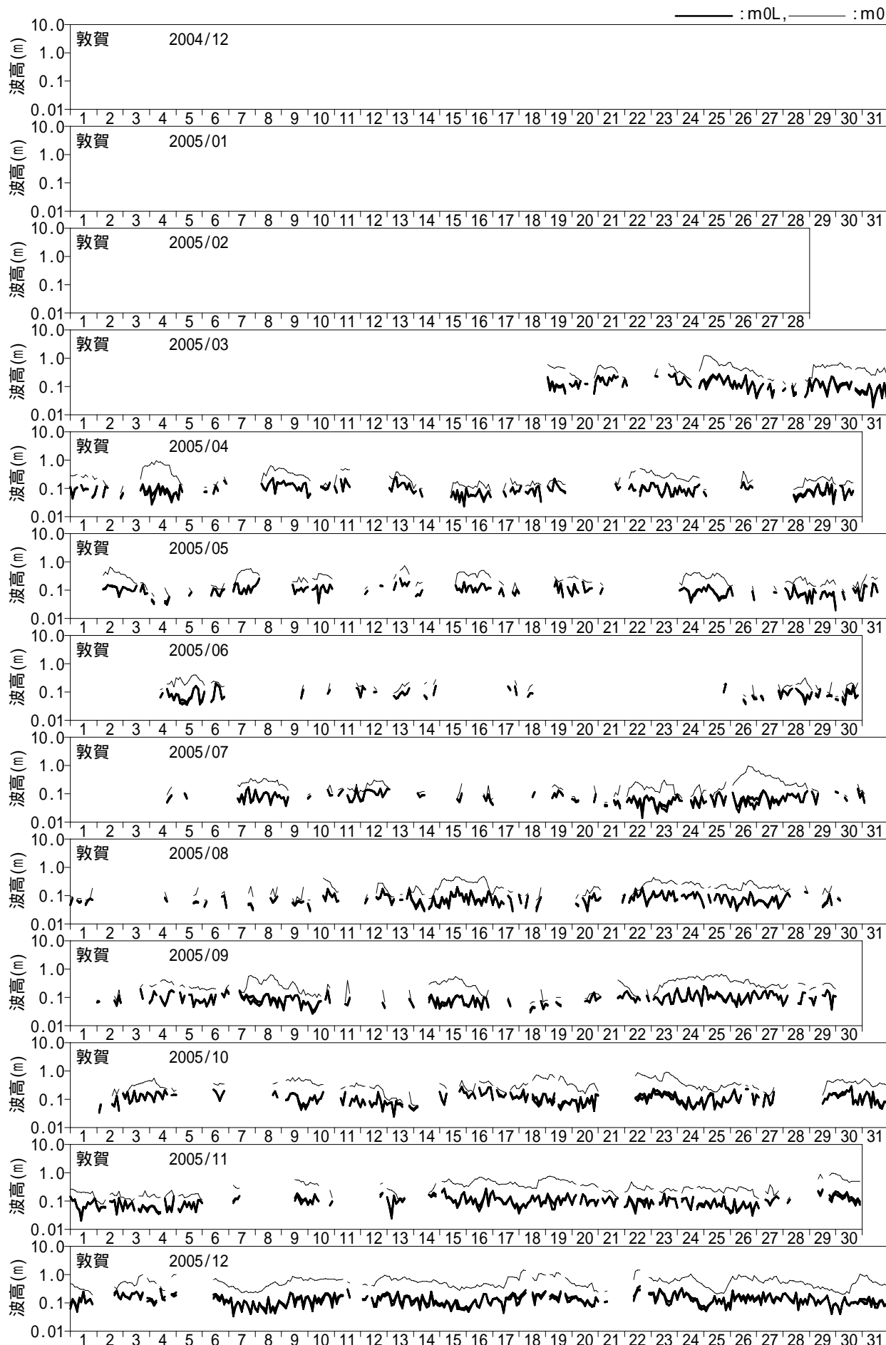
付図 - C.1.14 長周期波高の経時変化図 (敦賀)
