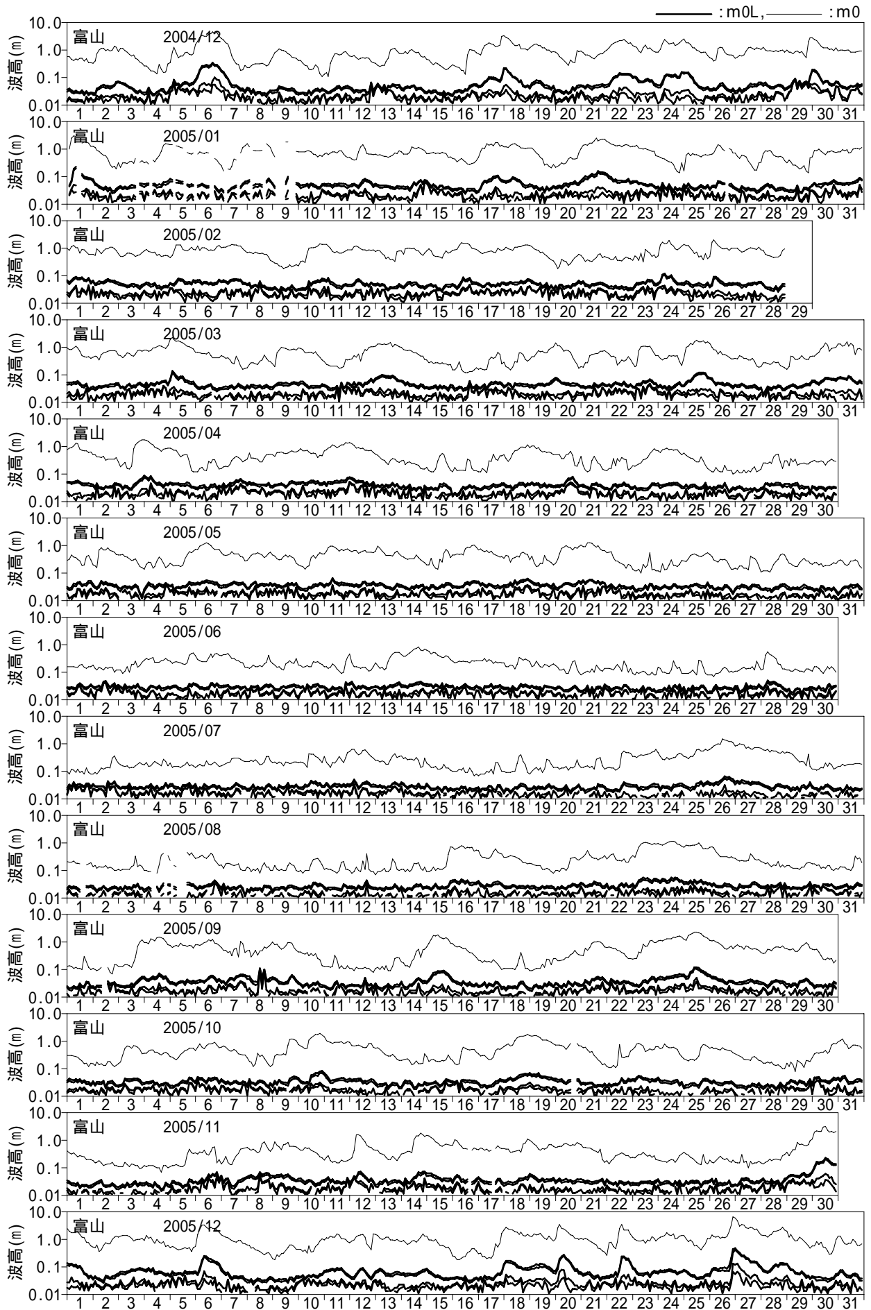
付図 - C.1.9 長周期波高の経時変化図 (富山)
