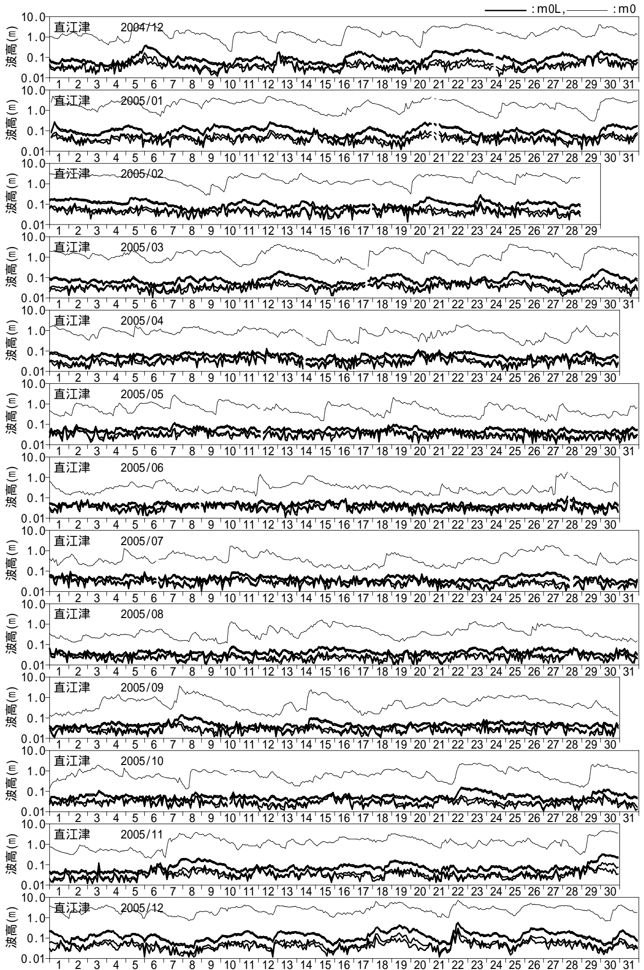
付図 - C.1.8 長周期波高の経時変化図 (直江津)
