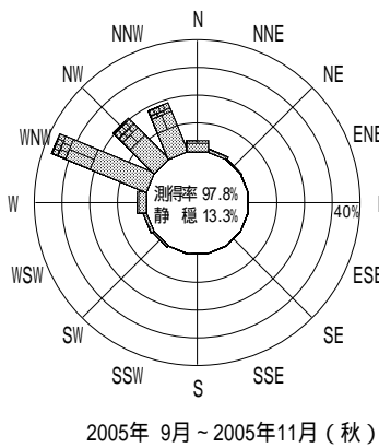
付図 - A.2.2 石狩新港 波高・波向別出現頻度図
