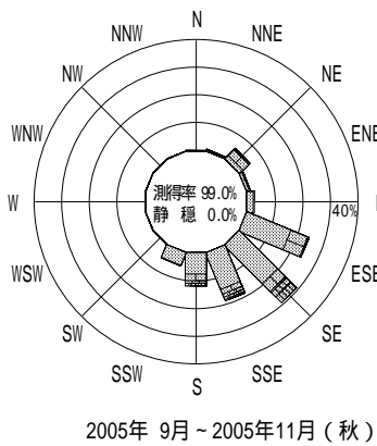
付図 - A.2.44 御前崎 波高・波向別出現頻度図
