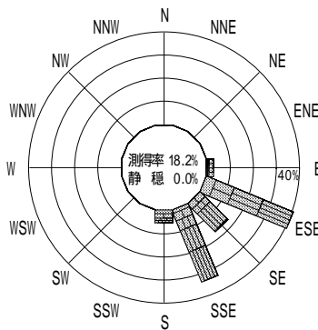
付図 - A.2.54 細島 波高・波向別出現頻度図
