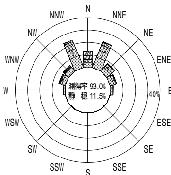
付図 - A.2.15 柴山 波高・波向別出現頻度図
