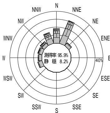
付図 - A.2.19 浜田 波高・波向別出現頻度図
