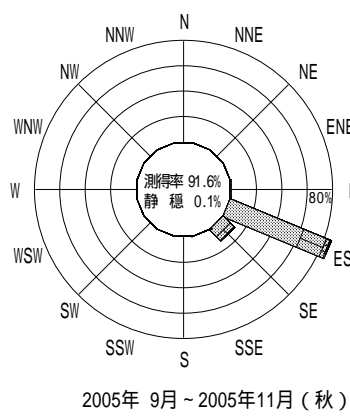
付図 - A.2.34 仙台新港 波高・波向別出現頻度図
