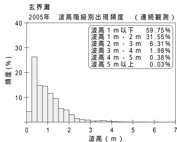
付図 - B.1.21 玄界灘 波候特性図 (连续観測)
