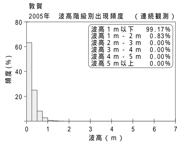
付図 - B.1.14 敦賀 波候特性図 (連続観測)
