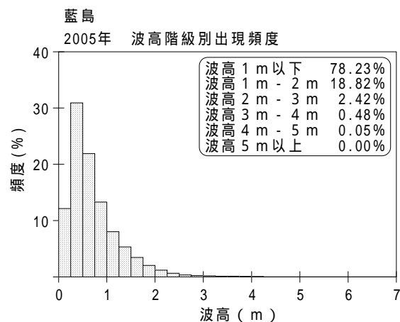
付図 - A.1.20 藍島 波候特性図
