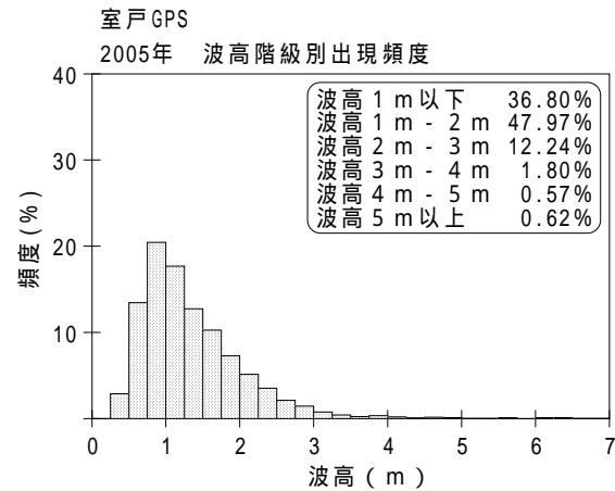
付図 - A.1.49 室戸GPS 波候特性図
