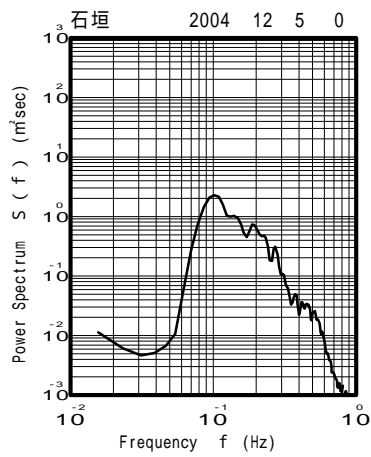
図 - 13.56 石垣 代表的な高波期間中のスペクトル
