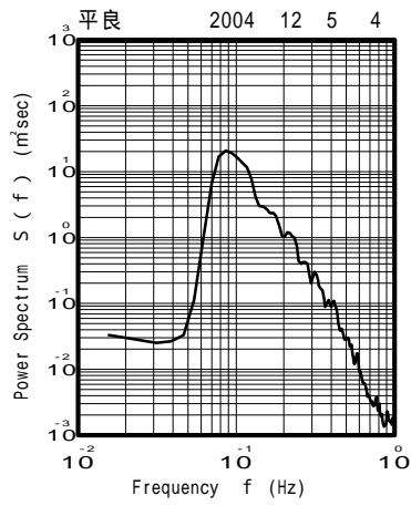
図 - 13.55 平良 代表的な高波期間中のスペクトル
