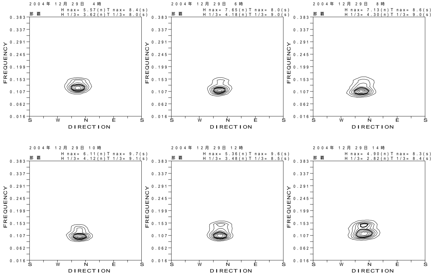
図 - 13.22 那覇 代表的な高波期間中の方向スペクトル
