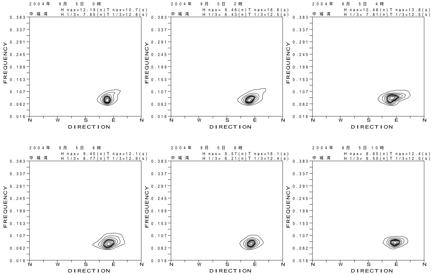
図 - 13.54 中城湾 代表的な高波期間中の方向スペクトル
