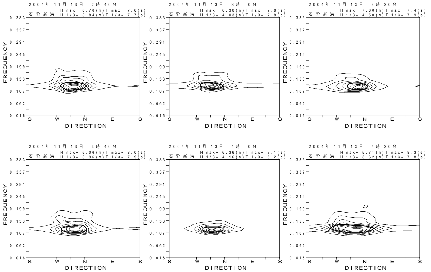
図 - 13.2 石狩新港 代表的な高波期間中の方向スペクトル
