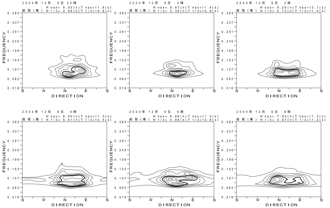
図 - 13.23 紋別(南) 代表的な高波期間中の方向スペクトル
