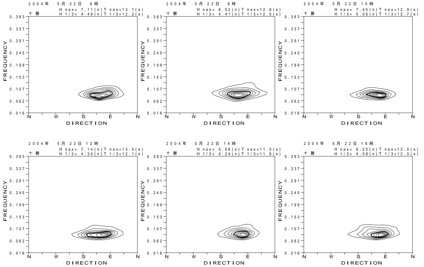
図 - 13.24 十勝 代表的な高波期間中の方向スペクトル
