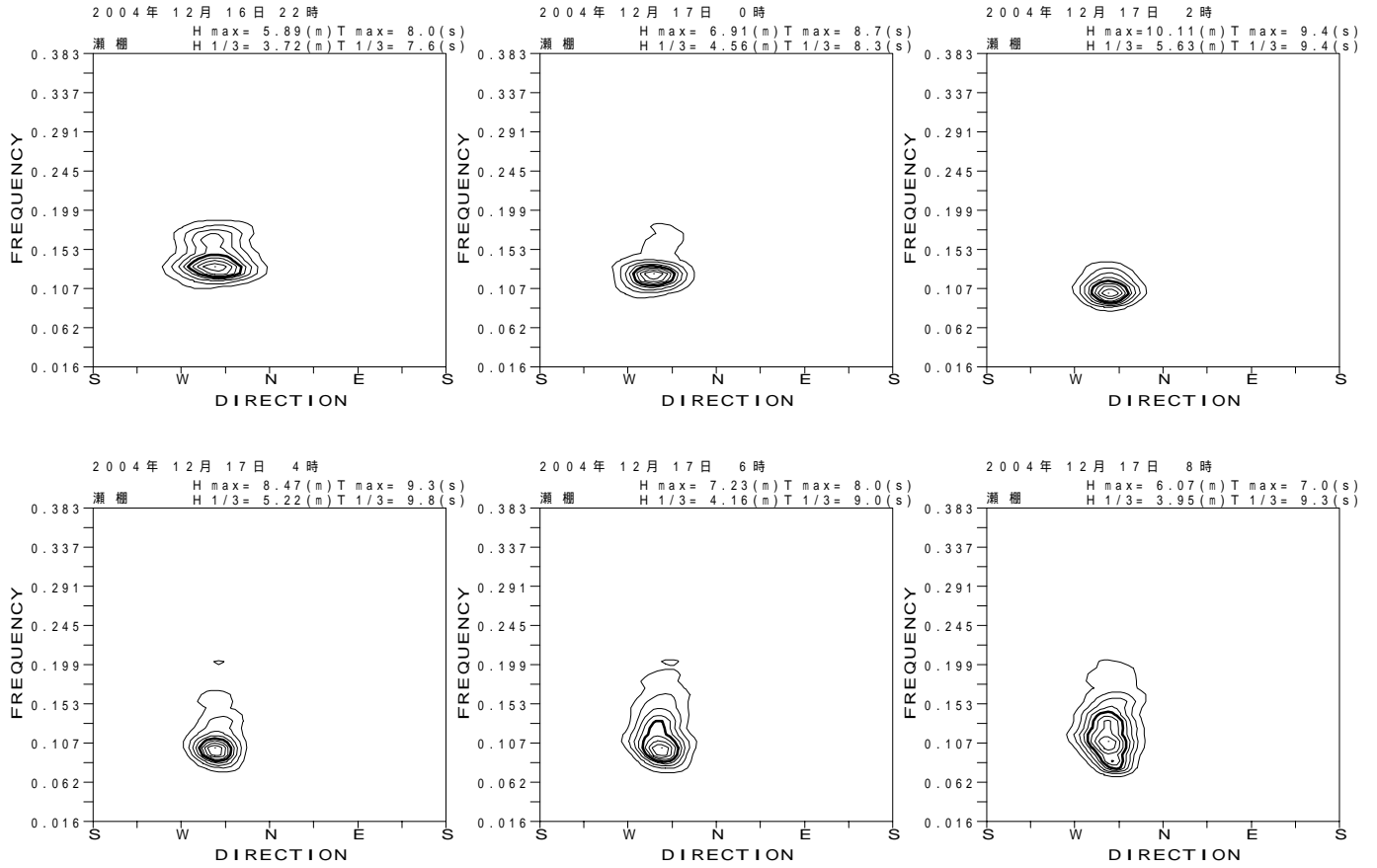
図 - 13.3 瀬棚 代表的な高波期間中の方向スペクトル
