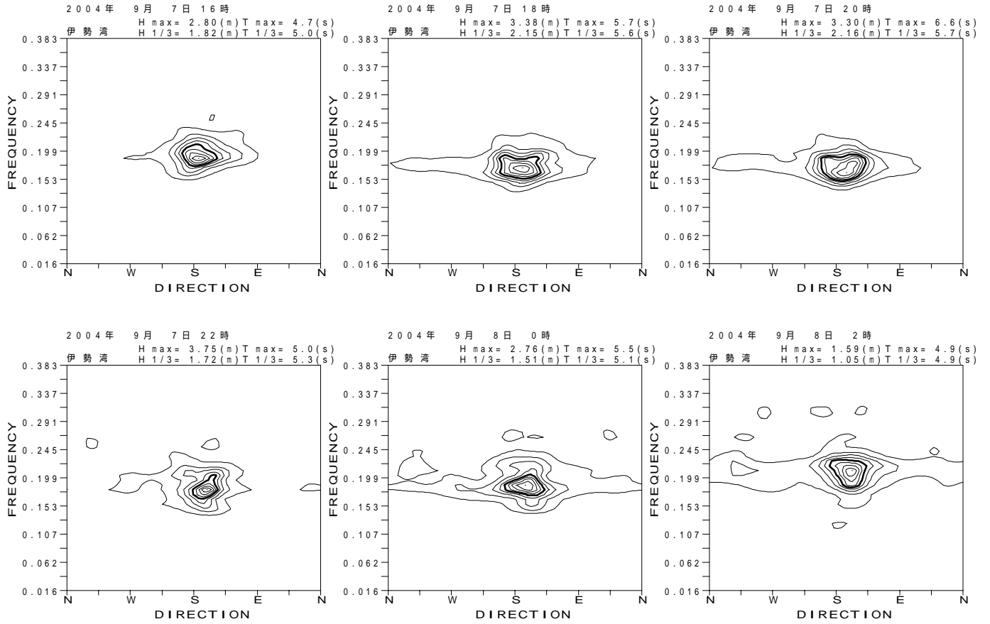
図 - 13.42 伊勢湾 代表的な高波期間中の方向スペクトル
