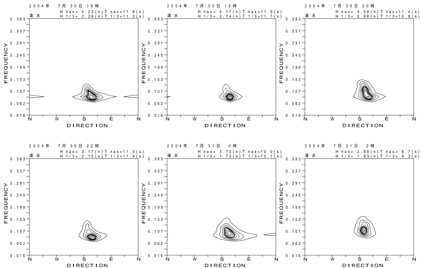
図 - 13.40 清水 代表的な高波期間中の方向スペクトル
