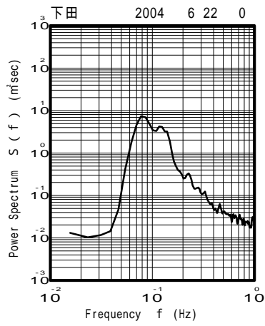
図 - 13.39 下田 代表的な高波期間中のスペクトル
