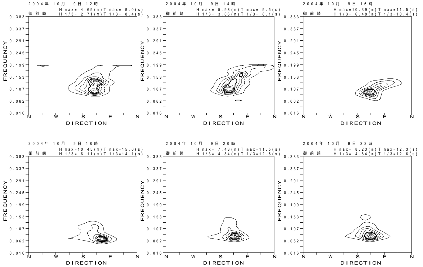
図 - 13.41 御前崎 代表的な高波期間中の方向スペクトル
