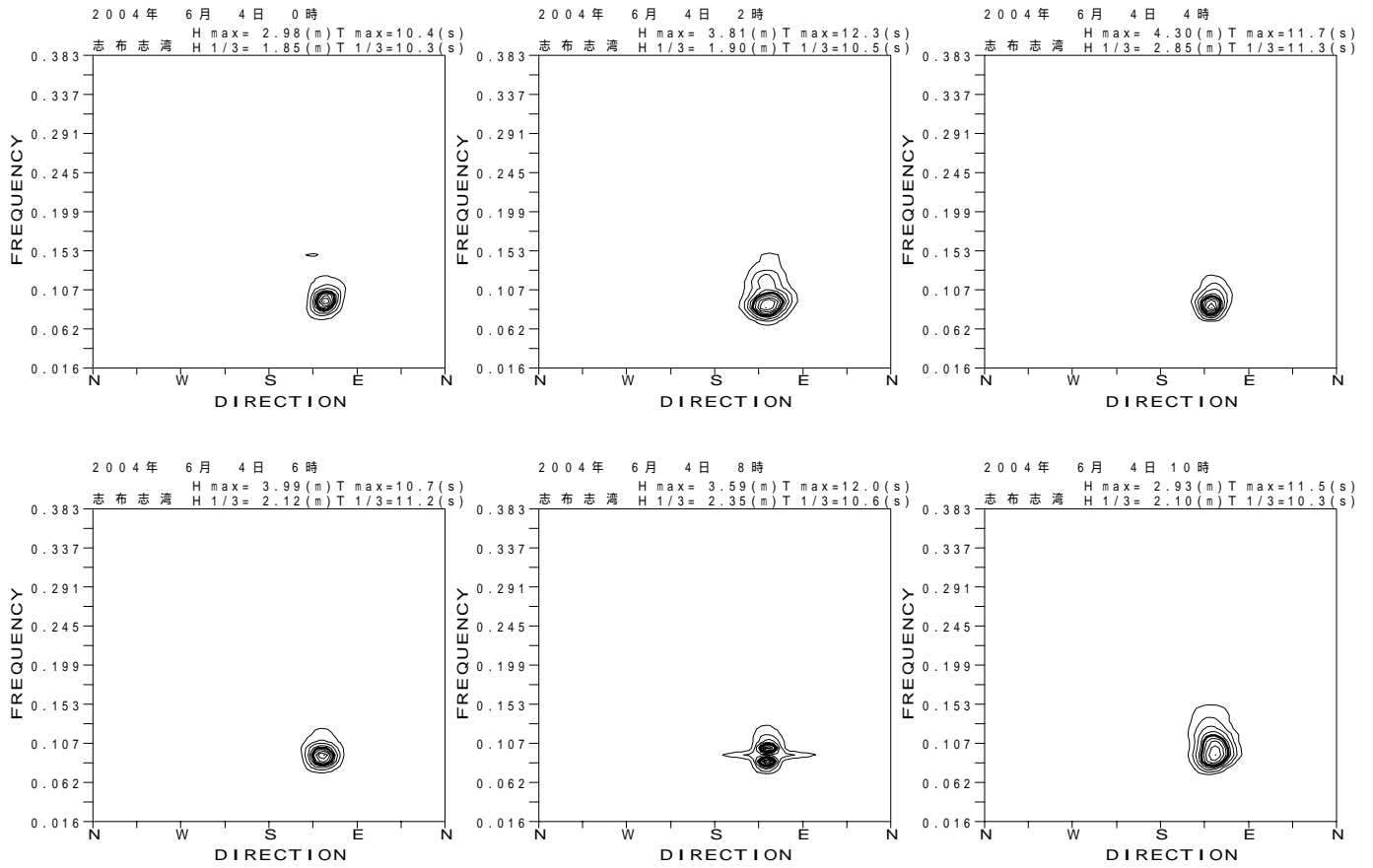
図 - 13.52 志布志湾 代表的な高波期間中の方向スペクトル
