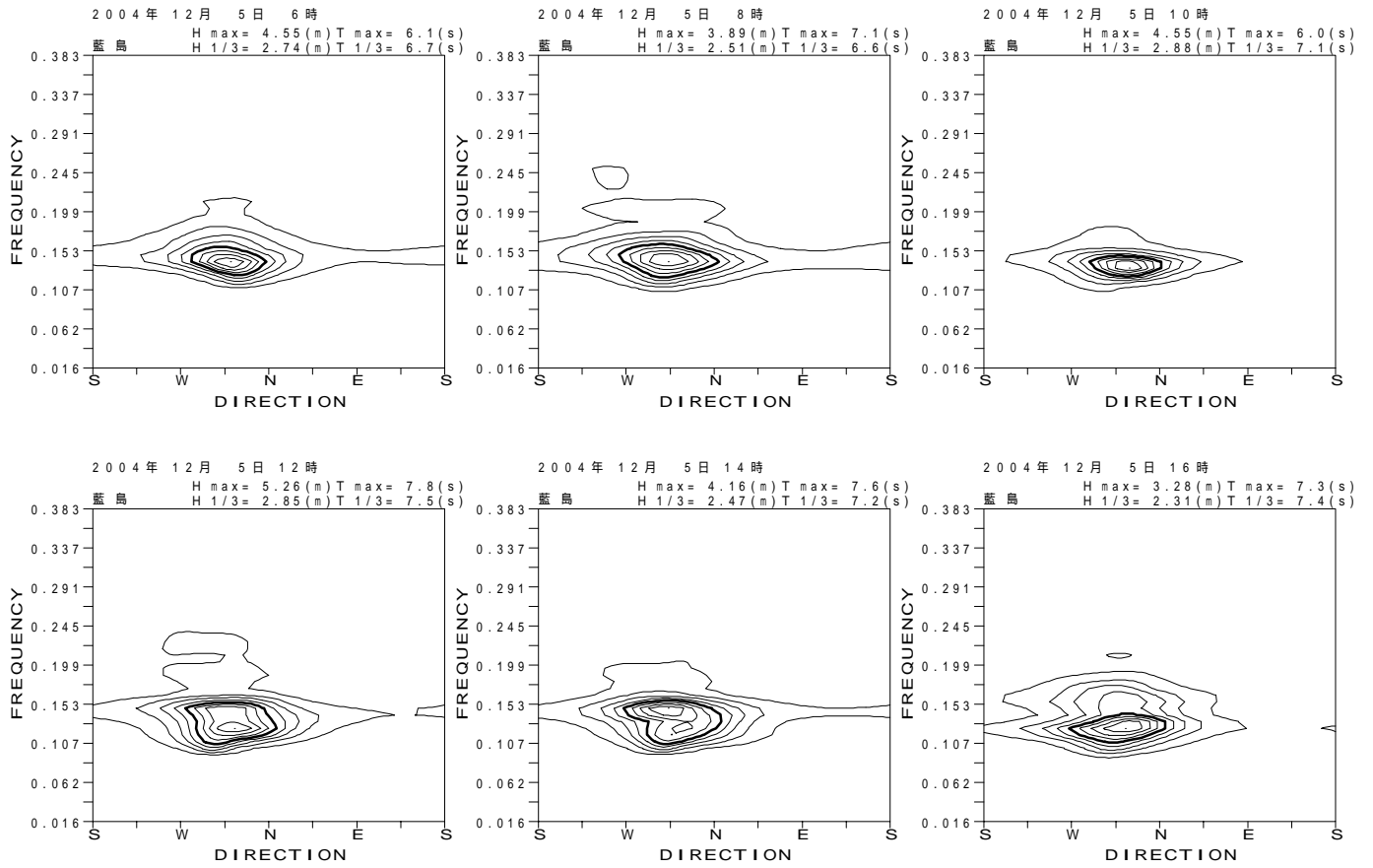
図 - 13.18 藍島 代表的な高波期間中の方向スペクトル
