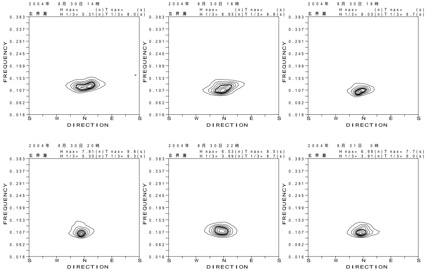
図 - 13.19 玄界灘 代表的な高波期間中の方向スペクトル
