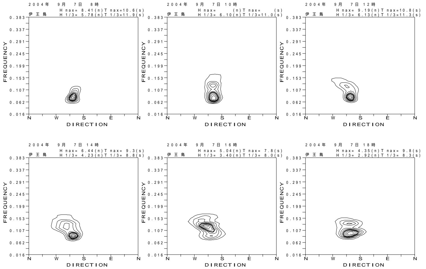
図 - 13.20 伊王島 代表的な高波期間中の方向スペクトル
