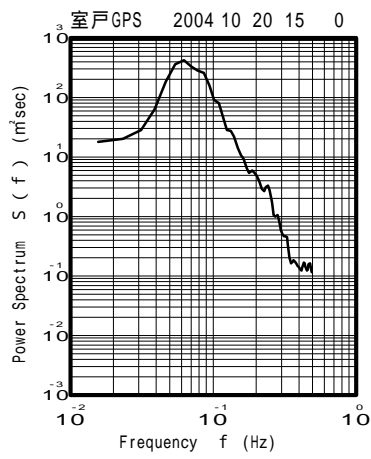
図 - 13.46 室戸GPS 代表的な高波期間中のスペクトル
