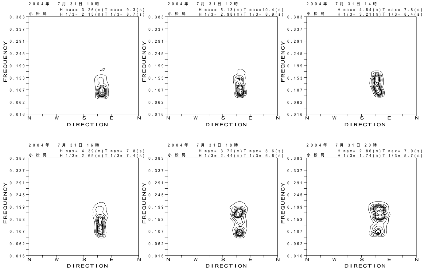
図 - 13.45 小松島 代表的な高波期間中の方向スペクトル
