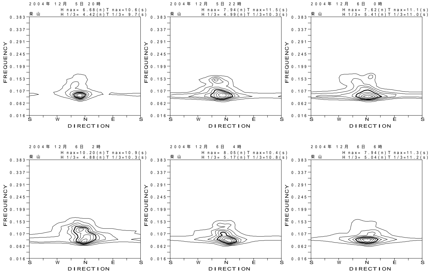
図 - 13.13 柴山 代表的な高波期間中の方向スペクトル
