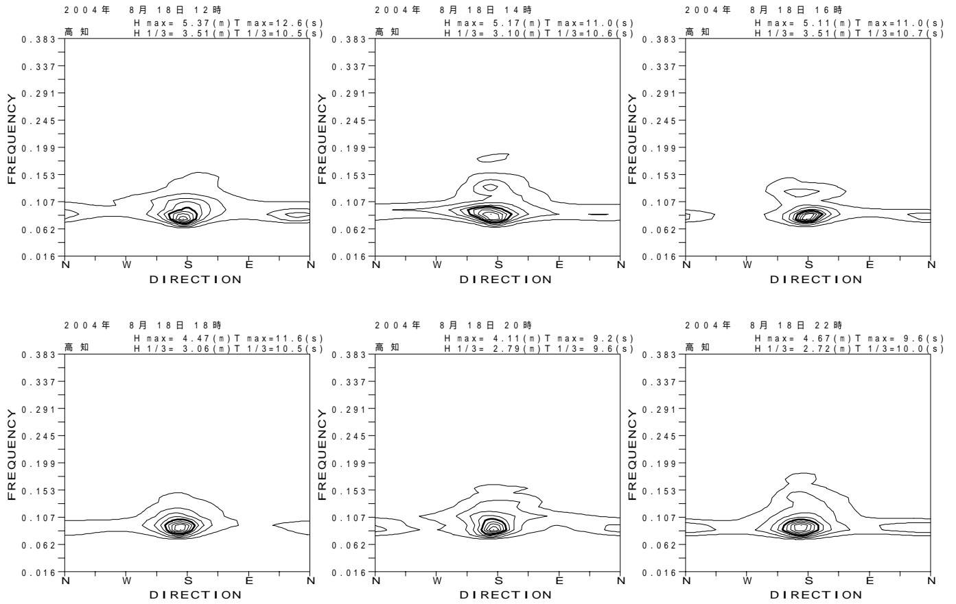
図 - 13.48 高知 代表的な高波期間中の方向スペクトル
