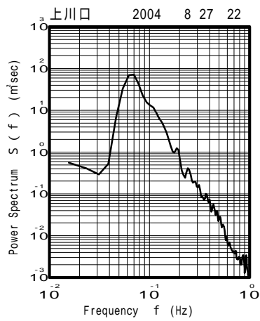
図 - 13.49 上川口 代表的な高波期間中のスペクトル
