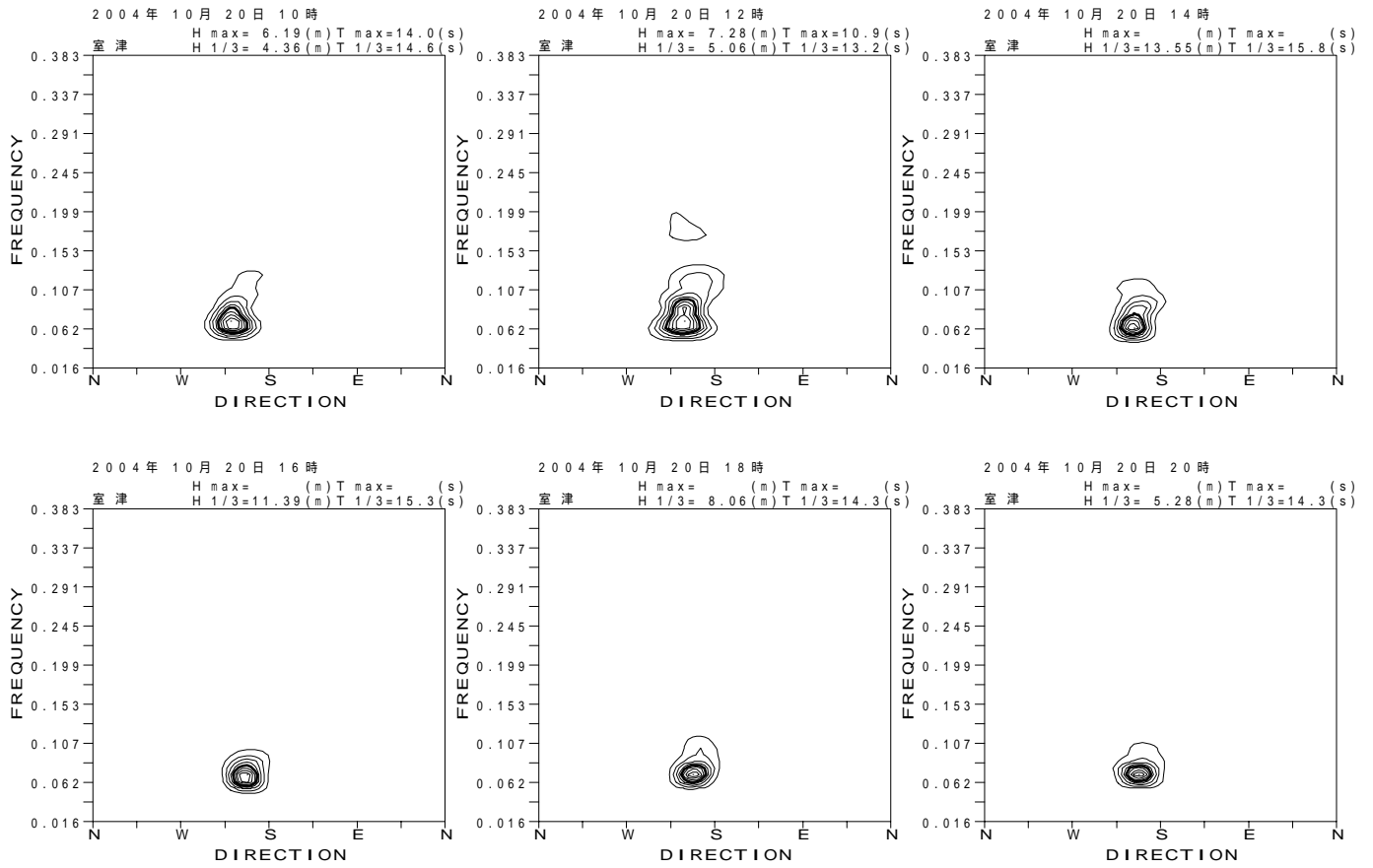
図 - 13.47 室津 代表的な高波期間中の方向スペクトル
