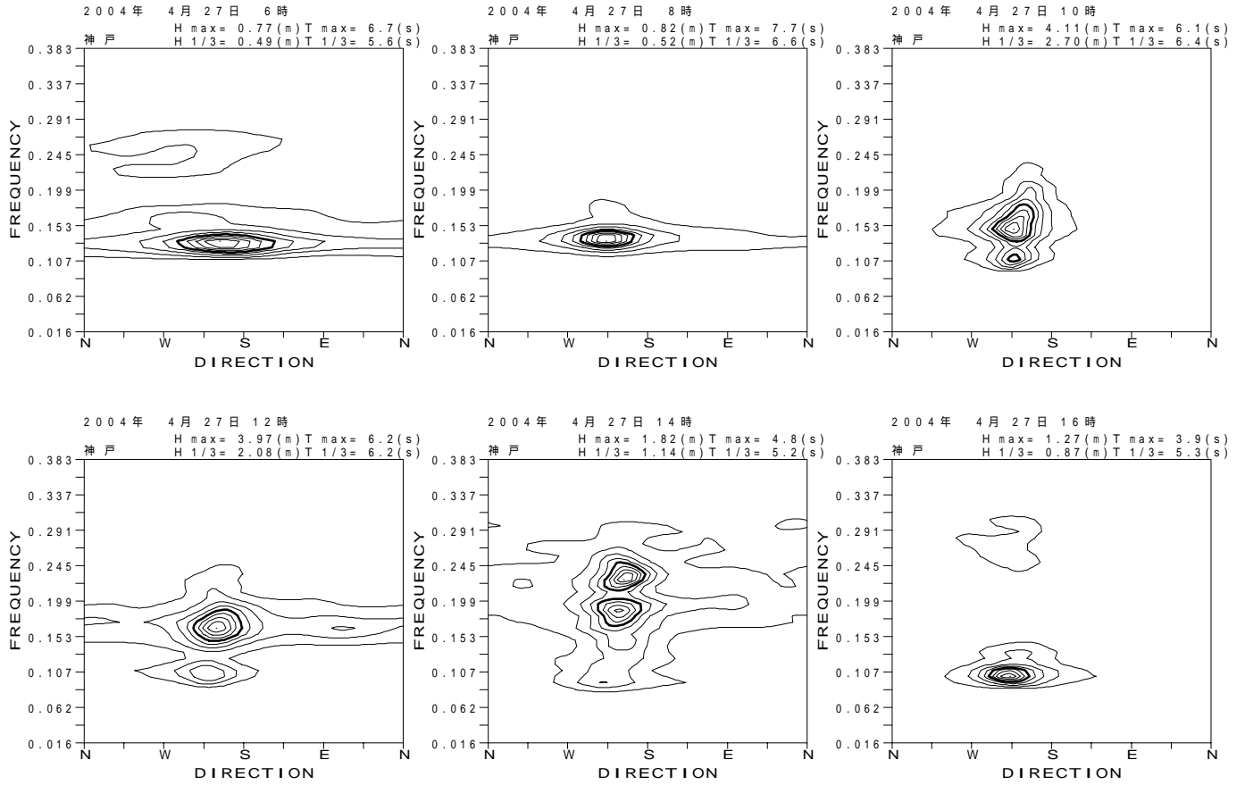
図 - 13.44 神戸 代表的な高波期間中の方向スペクトル
