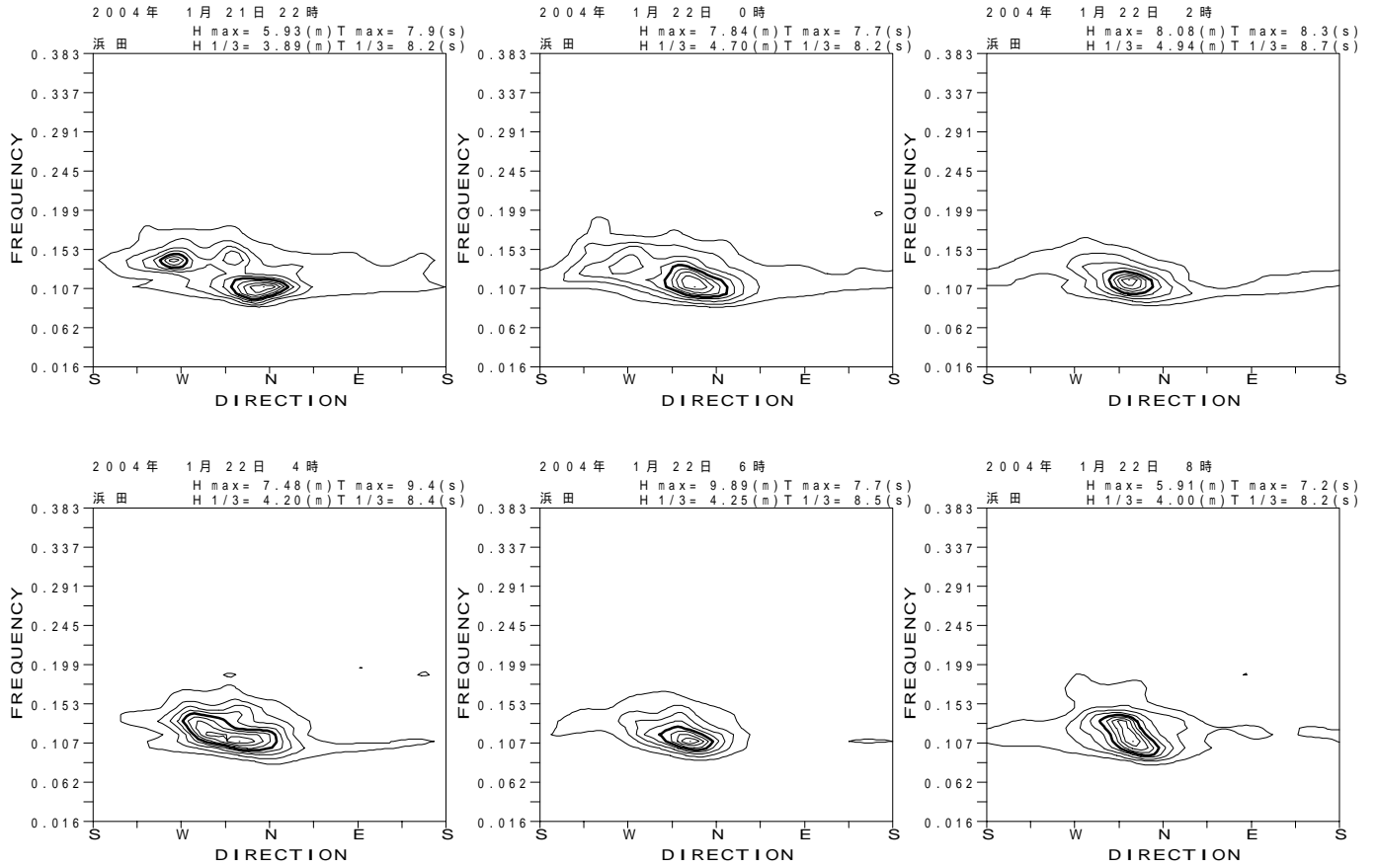
図 - 13.17 浜田 代表的な高波期間中の方向スペクトル
