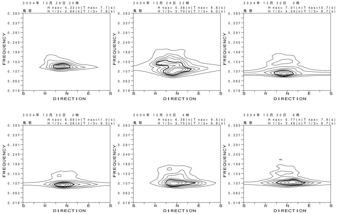
図 - 13.15 鳥取 代表的な高波期間中の方向スペクトル
