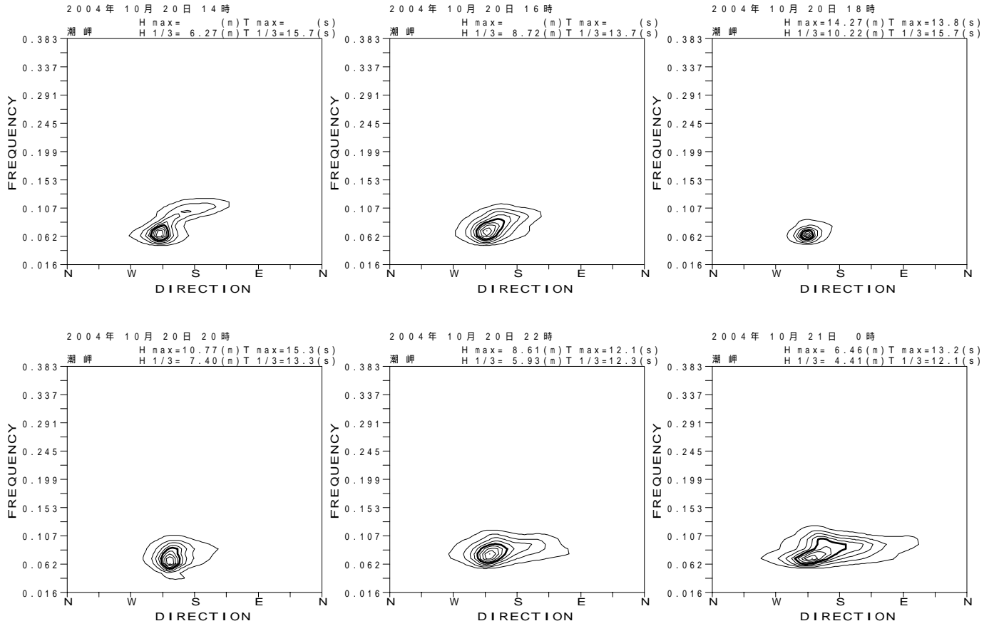
図 - 13.43 潮岬 代表的な高波期間中の方向スペクトル
